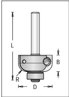
T.C. Blade 3112006
